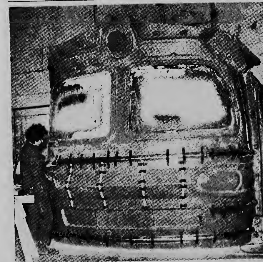
Despues cu nan a hasi exitoso uso di fiberglass/Duroplast pa caroseria di autonon, nan kier usa e material aki tambe pa locomotoran electrico na Checoslovakia. Aki nos ta mira, un prototipo pa un capa di un locomotora.
